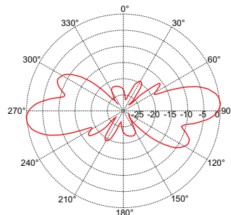
Bidirecional polarização vertical (Plano E)
