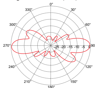
Omnidirecional polarização vertical (Plano E)
