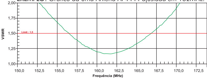
EXEMPLO: Gráfico da uma Antena AP4444 ajustada em 162MHz.
