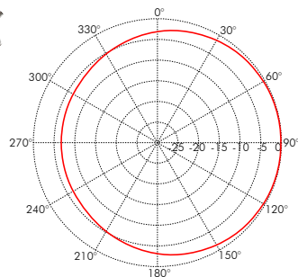
Offset de polarización horizontal (plano H)
