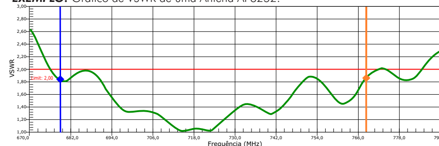
EXEMPLO: Gráfico de VSWR de uma Antena AP8252.
